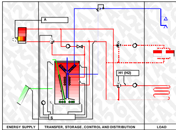
Abb. 11: System mit drucklosem Speicher und thermosyphonisch betriebenen Wärmetauschern
