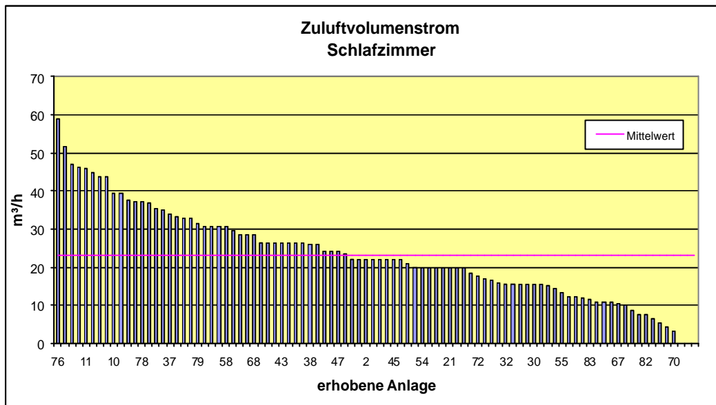
Abbildung 4: Erhobene Zuluftvolumenströme im Schlafzimmer bei Normalbetriebsstufe (Basis: 92 Anlagen; Die rosa Linie stellt den Mittelwert über alle untersuchten Anlagen dar.)
