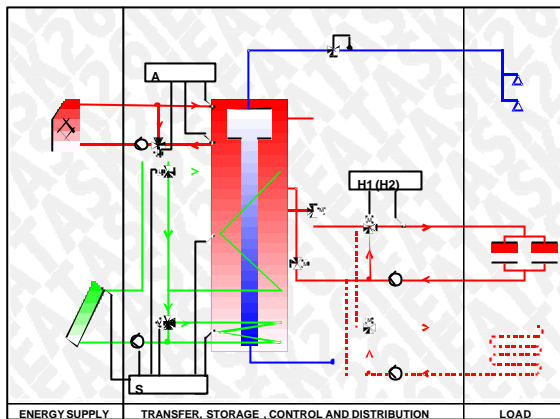
Abb. 9: Tank in Tank System für hohe solare Deckungsgrade
