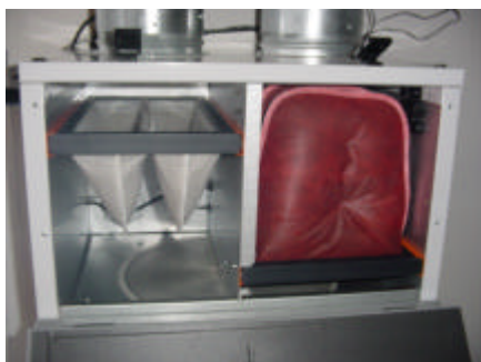
Abbildung 10: Lüftungsgerät mit Taschenfiltern auf der Zu- und Abluftseite
