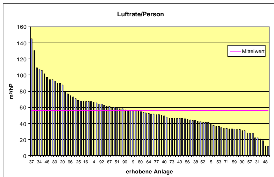
Abbildung 3: Frischluftvolumenstrom pro Person bei Normalbetriebsstufe (Basis: 92 Anlagen; Die rosa Linie stellt den Mittelwert über alle untersuchten Anlagen dar.)
