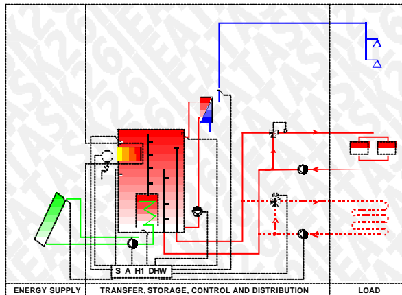
Abb. 12: Kompaktanlage mit speicherintegriertem Gasbrenner und Schichtenladern
