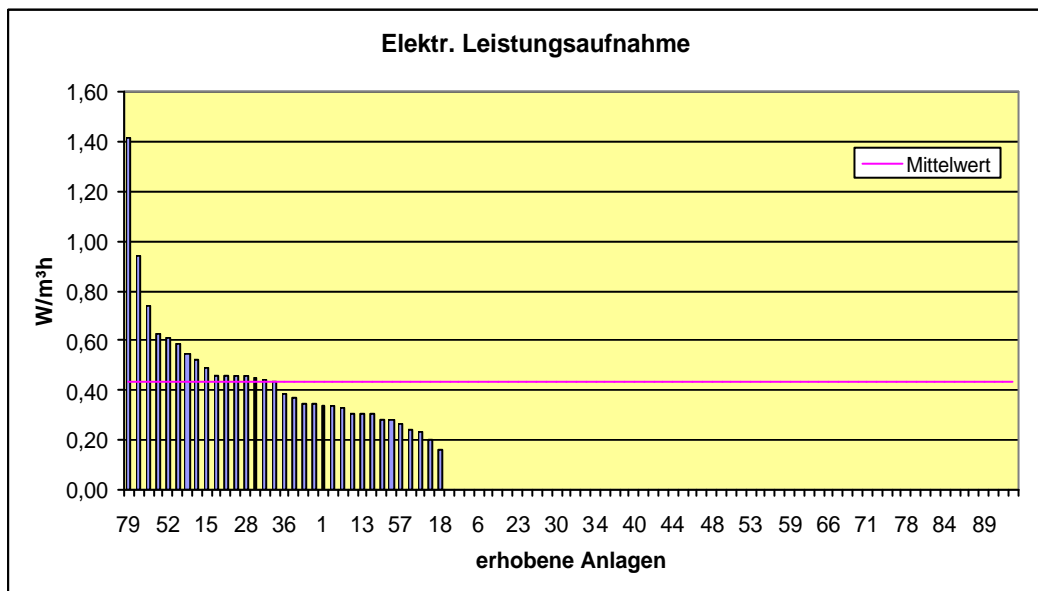
Abbildung 9: Elektr. Leistungsaufnahme der Gesamtanlage
