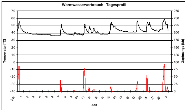
Abb. 3: Warmwas-serbedarf in einem Ein-familienhaus: Tageszapf-profil
