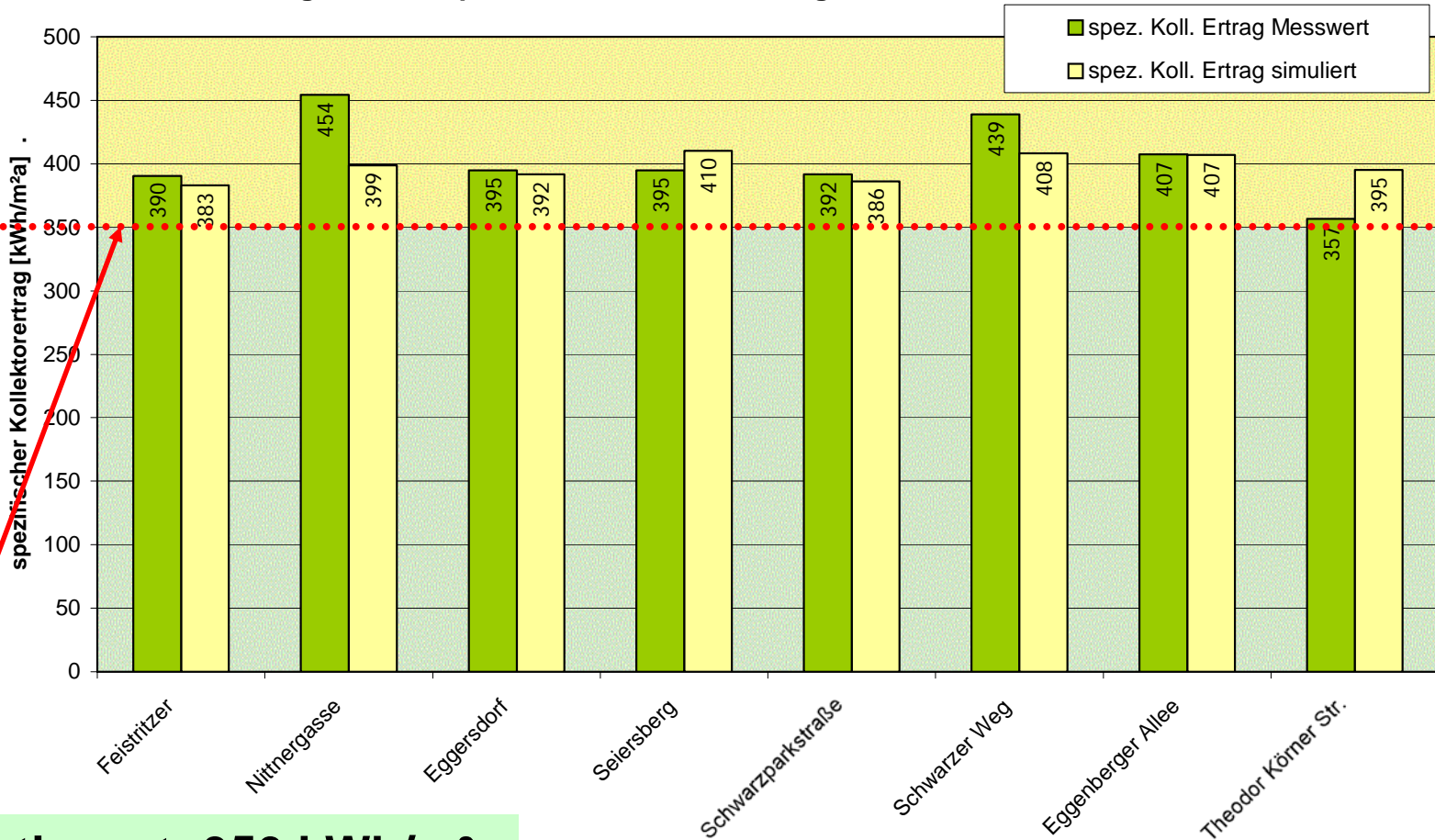
Vergleich der spezifischen Kollektorerträge - Simulation mit Messwert
